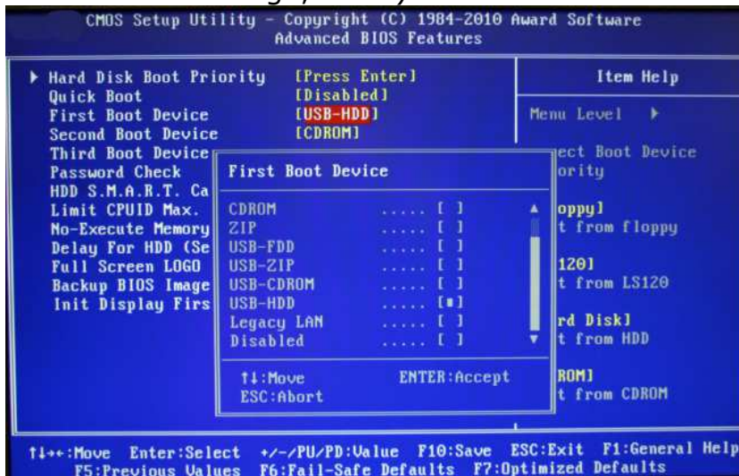
Interface utilisateur d'un BIOS Award
